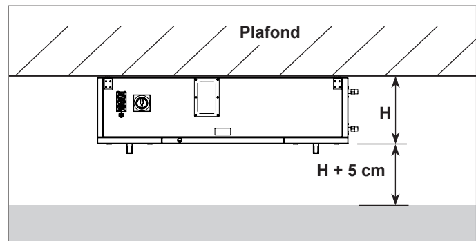
Fig. 5: FHX plafondmontage / minima- le afstand voor onderhouds- werkzaamheden
