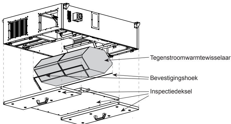
Afb.24: Demontage tegenstroomwarmtewisselaar
