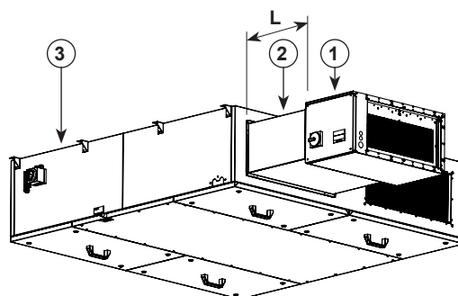
Fig. 22: Aansluiten EHM op FHX 1600/2400
