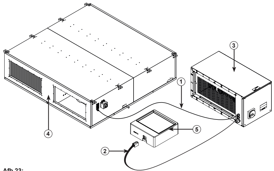
Afb.23: Aansluiting van de bedieningseenheid op de verwarmingsmodule
