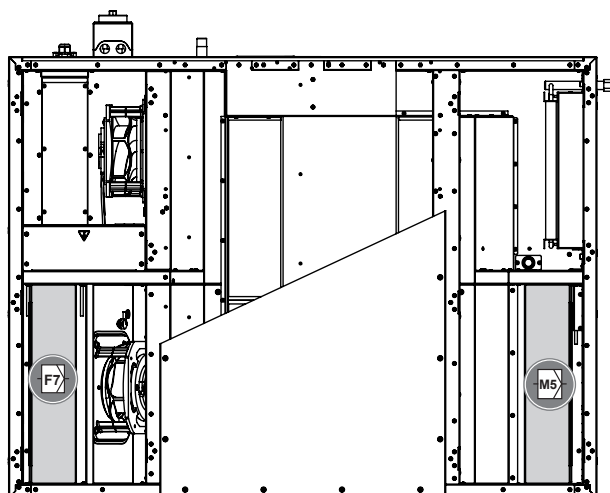
Afb.25: Positie luchtfilter
