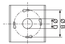
Afb.29a: Montageafmetingen van het bedieningspaneel.
