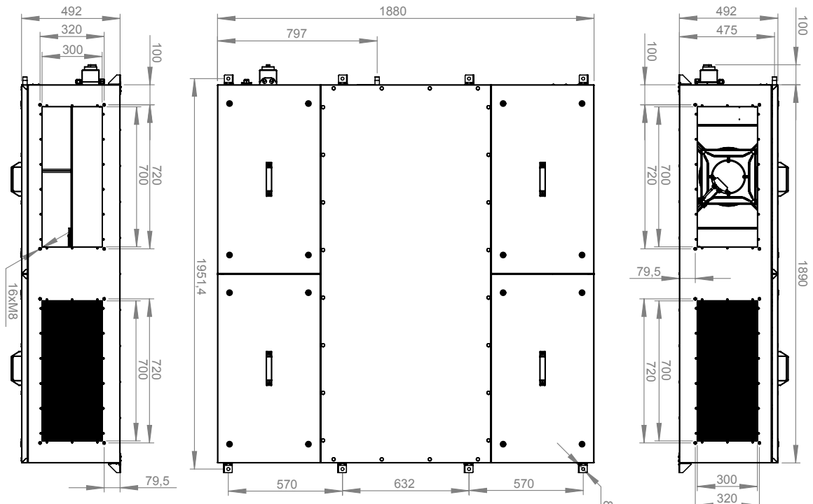
FHX 2400
