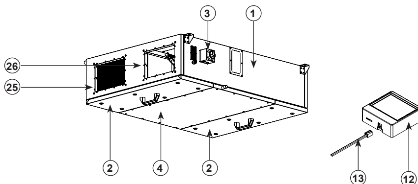
Afb.1 FHX 600
