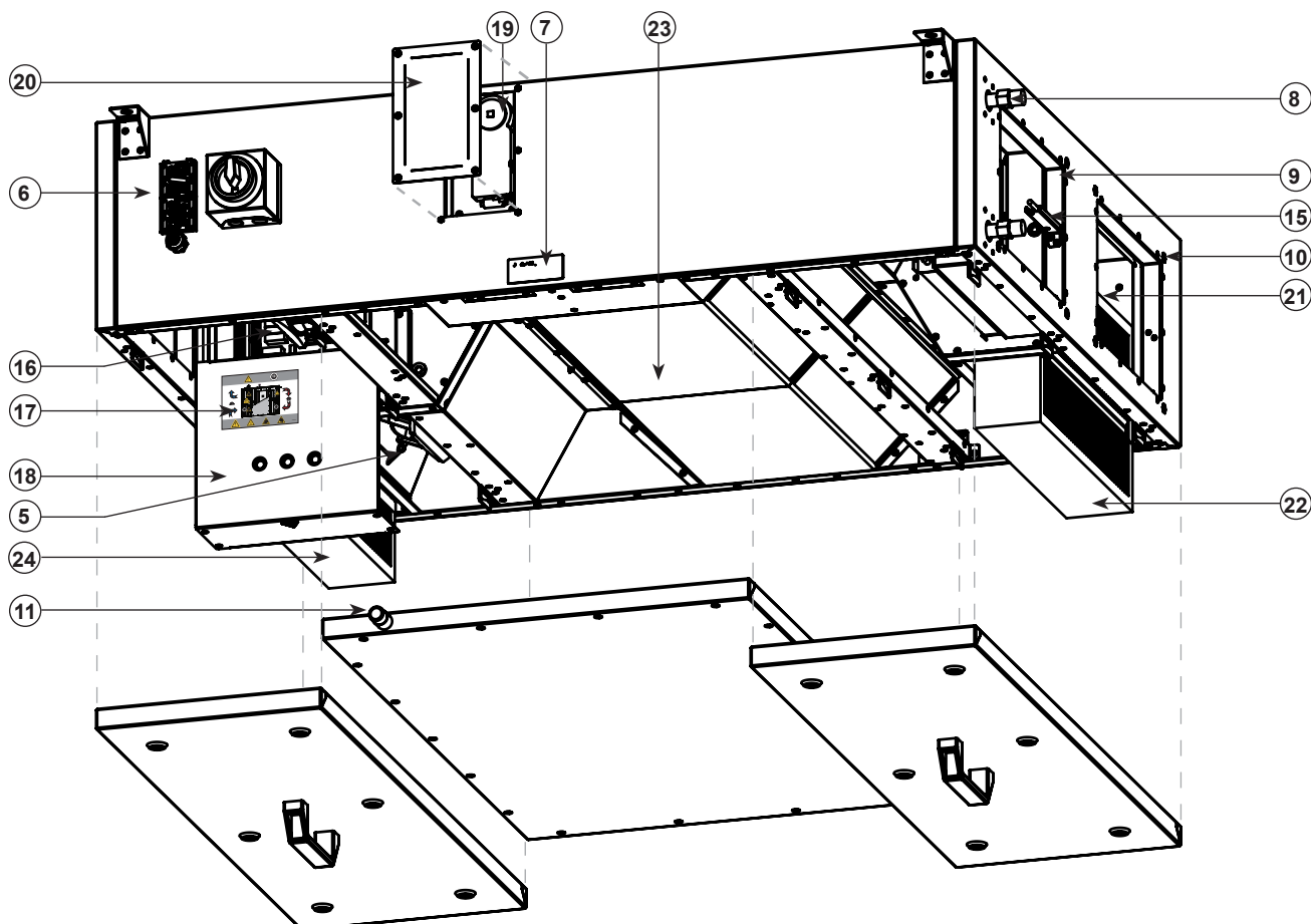
Afb.2: FHX 600
