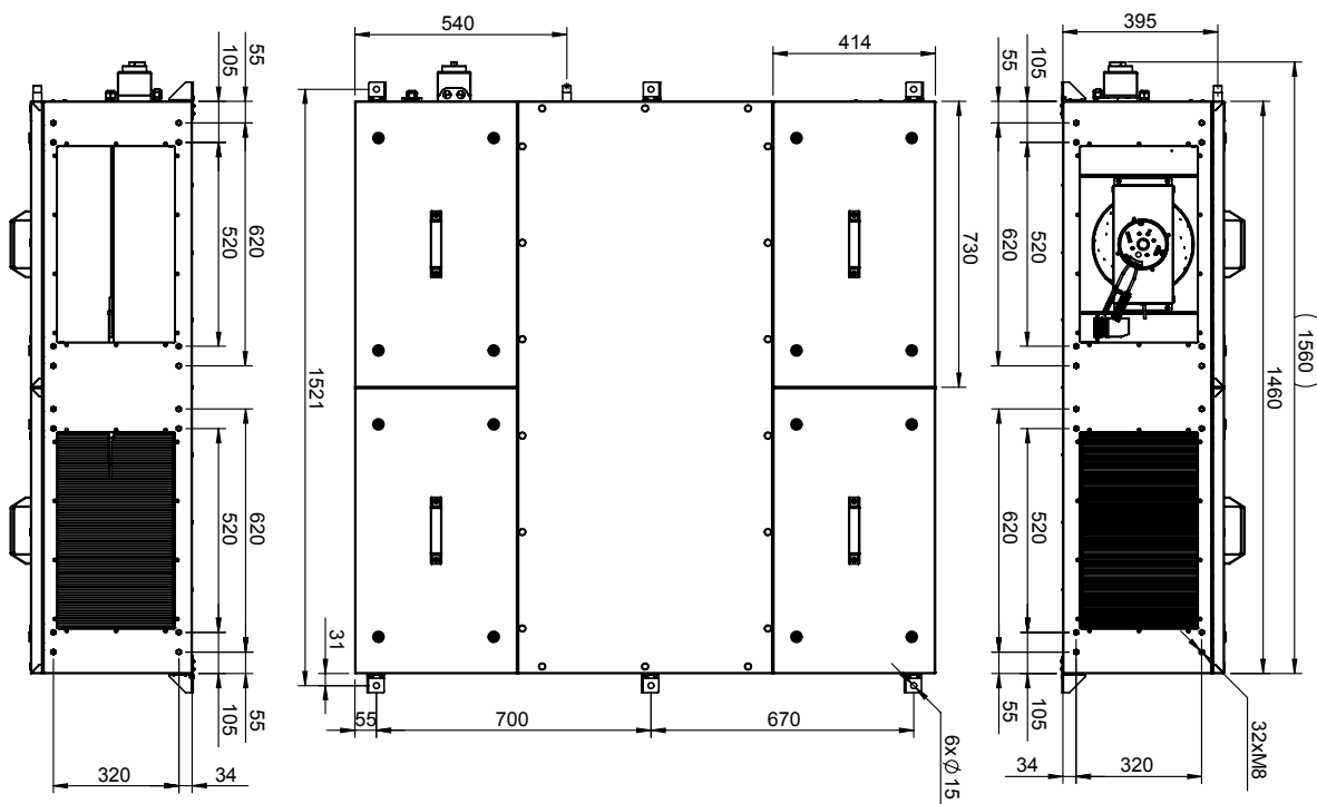
FHX 1200
