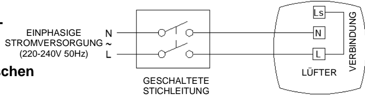
Abb.2 Konstanter Boost ohne Leerlauf-Funktion (T, HT)
