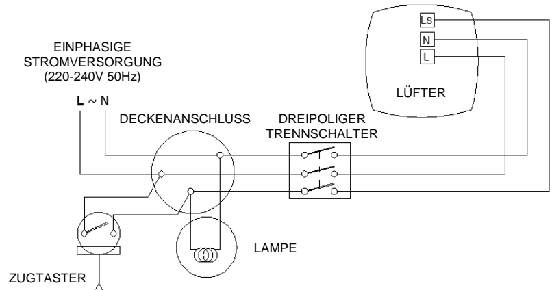
Abb.4 Konstanter Leerlauf mit Boost-Funktion über Fernschalter. (T, HT)
